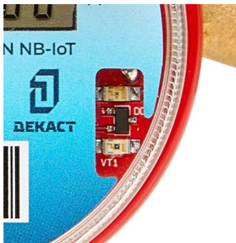
Рисунок 10 — Оптический порт
